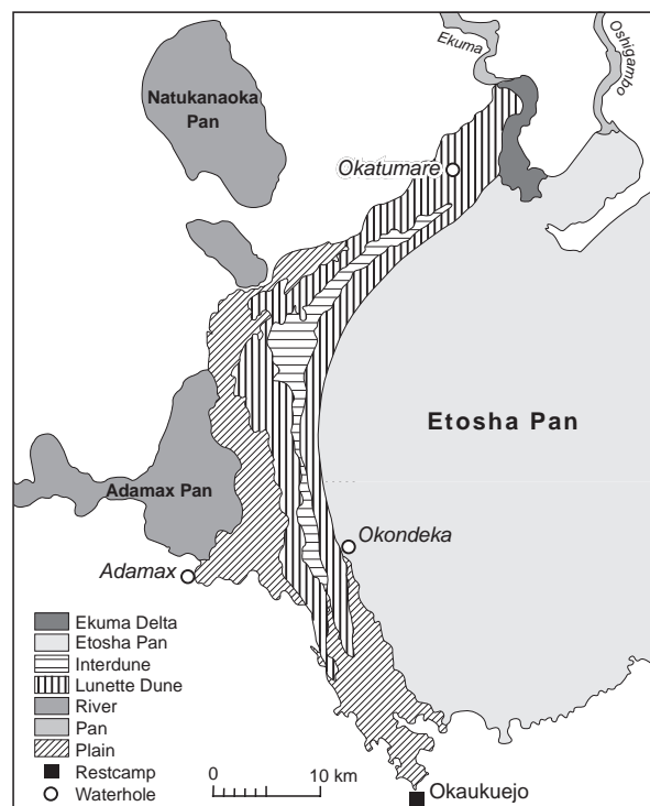
Fig. 2: Principal Geomorphological Units of the Study Area. Geomorphologische Einteilung des Untersuchungsgebiets.
